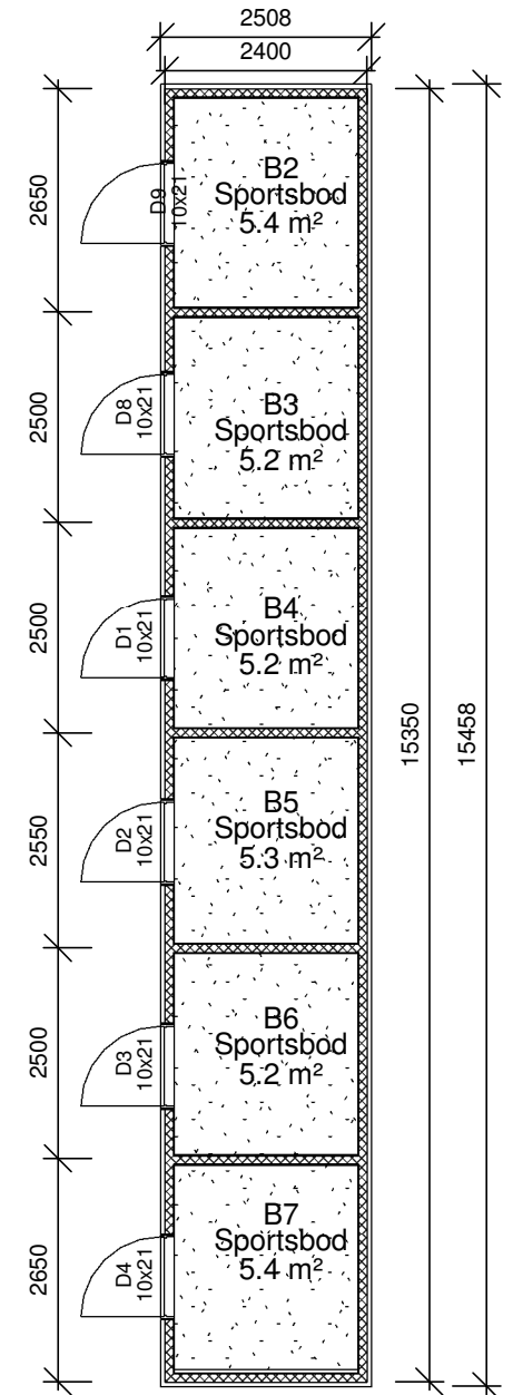
1.0 - 1.etasje 1 : 100
