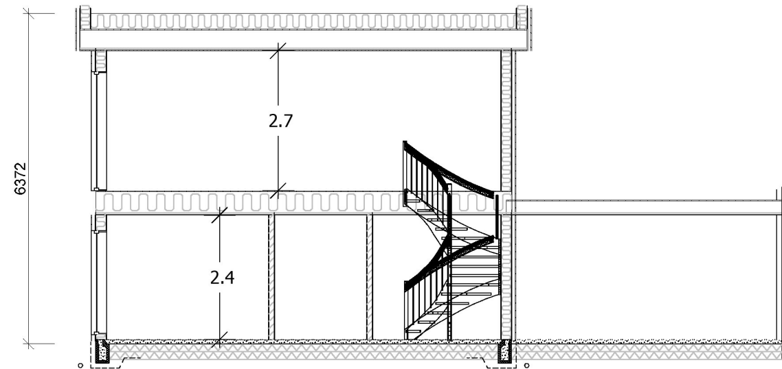
Snitt A:A
