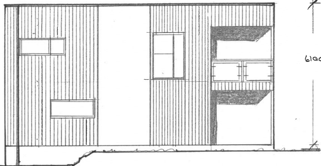
FASADE VEST
