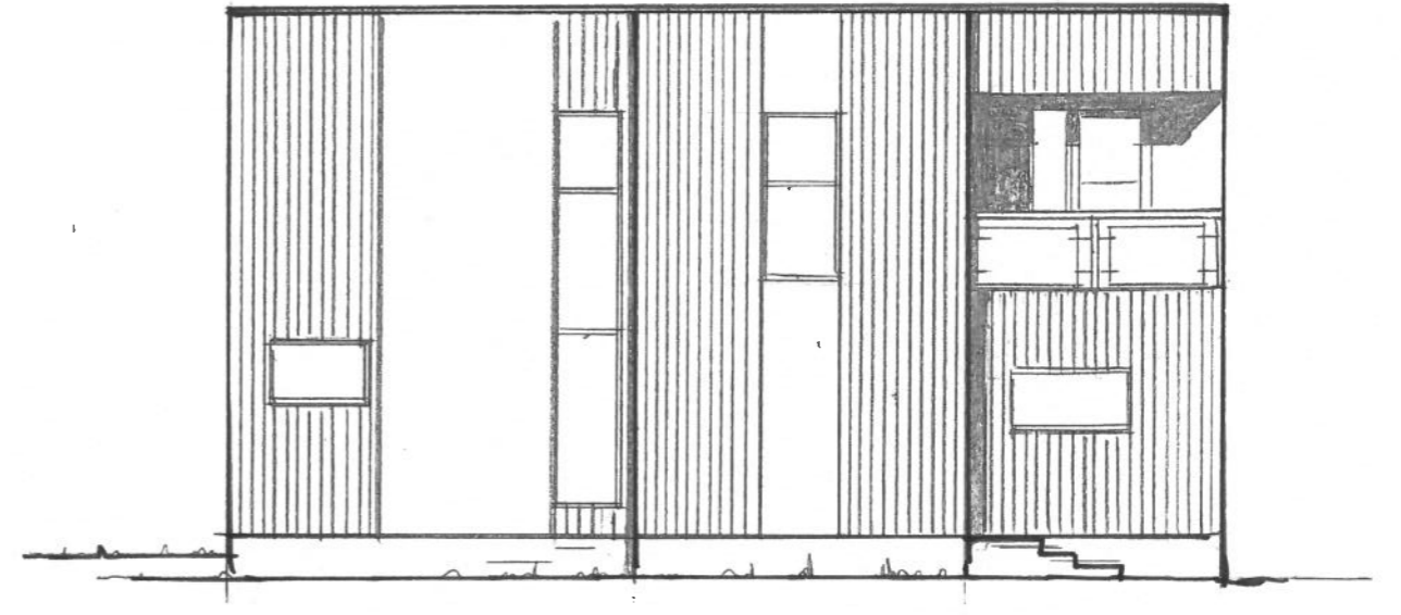
FASADE ØST
