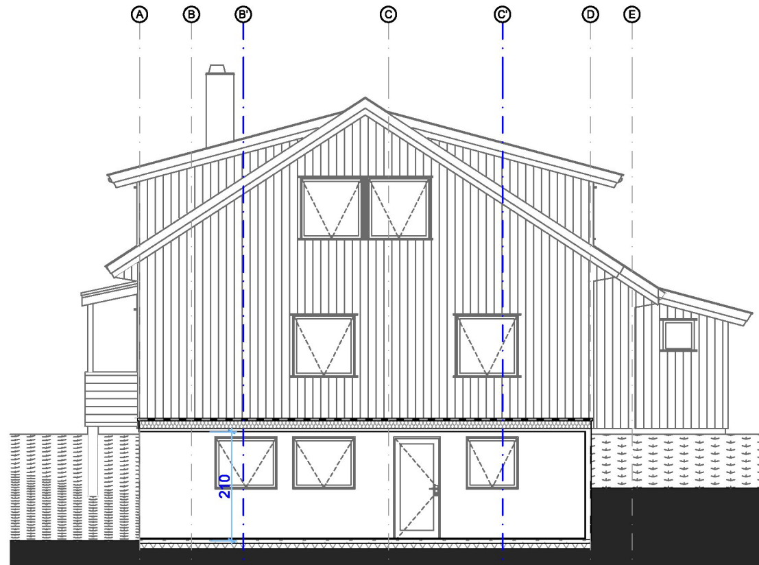
SNITT B-B
