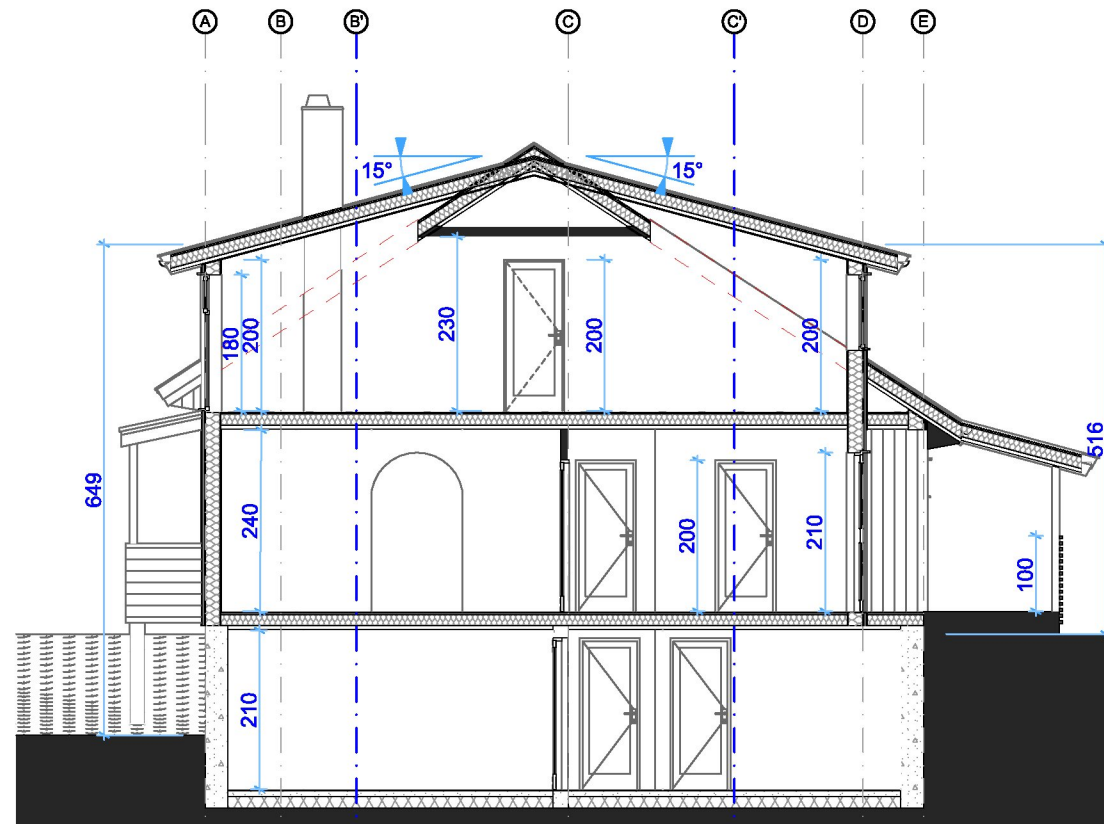
SNITT C-C
