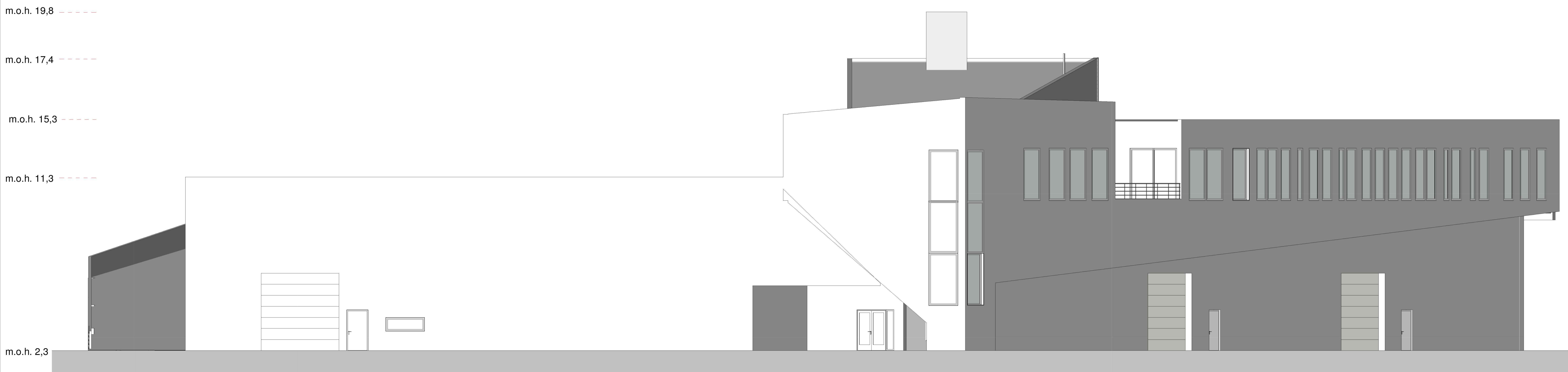
Fasade Vest 1 : 100
