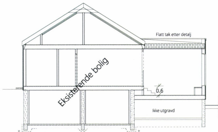
Snitt A-A
