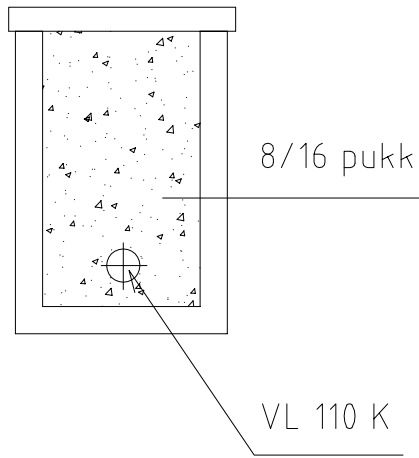
Tverrsnitt kulvert Lengde 5m
