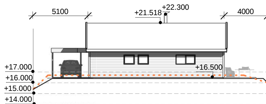
Vest TS 1 : 200
