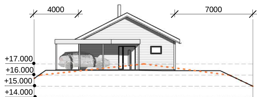
Nord TS 1 : 200
