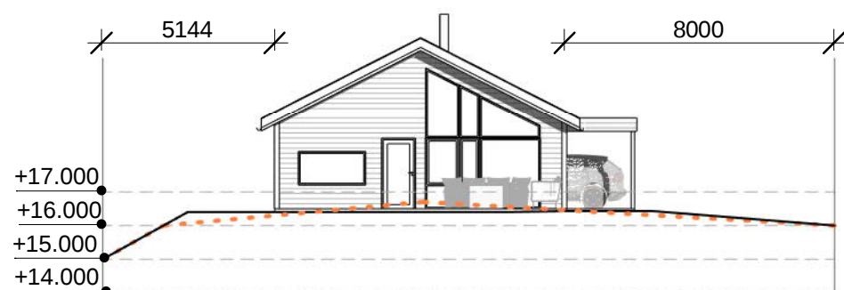
Sør TS 1 : 200
