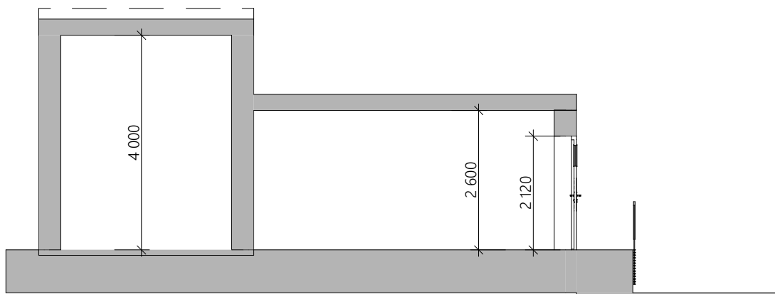
1:100 Snitt A
