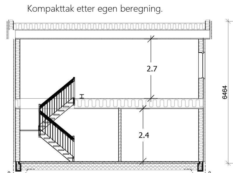
Snitt A:A
