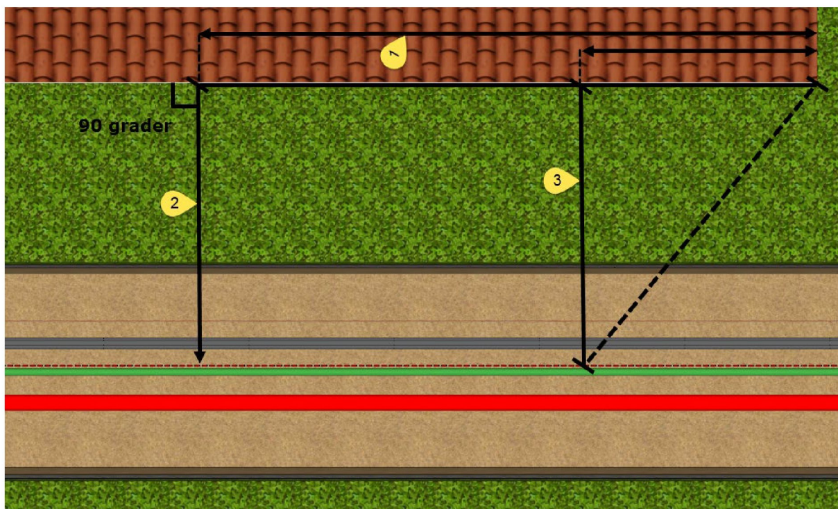
Figur 14 RT8513 - Prinsippkisse for mål
