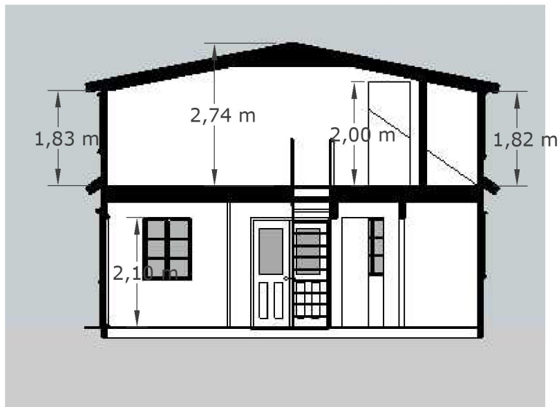
Snitt Vest
