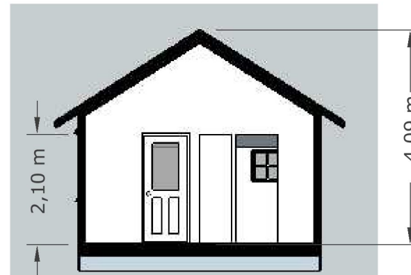
Snitt Kortside
