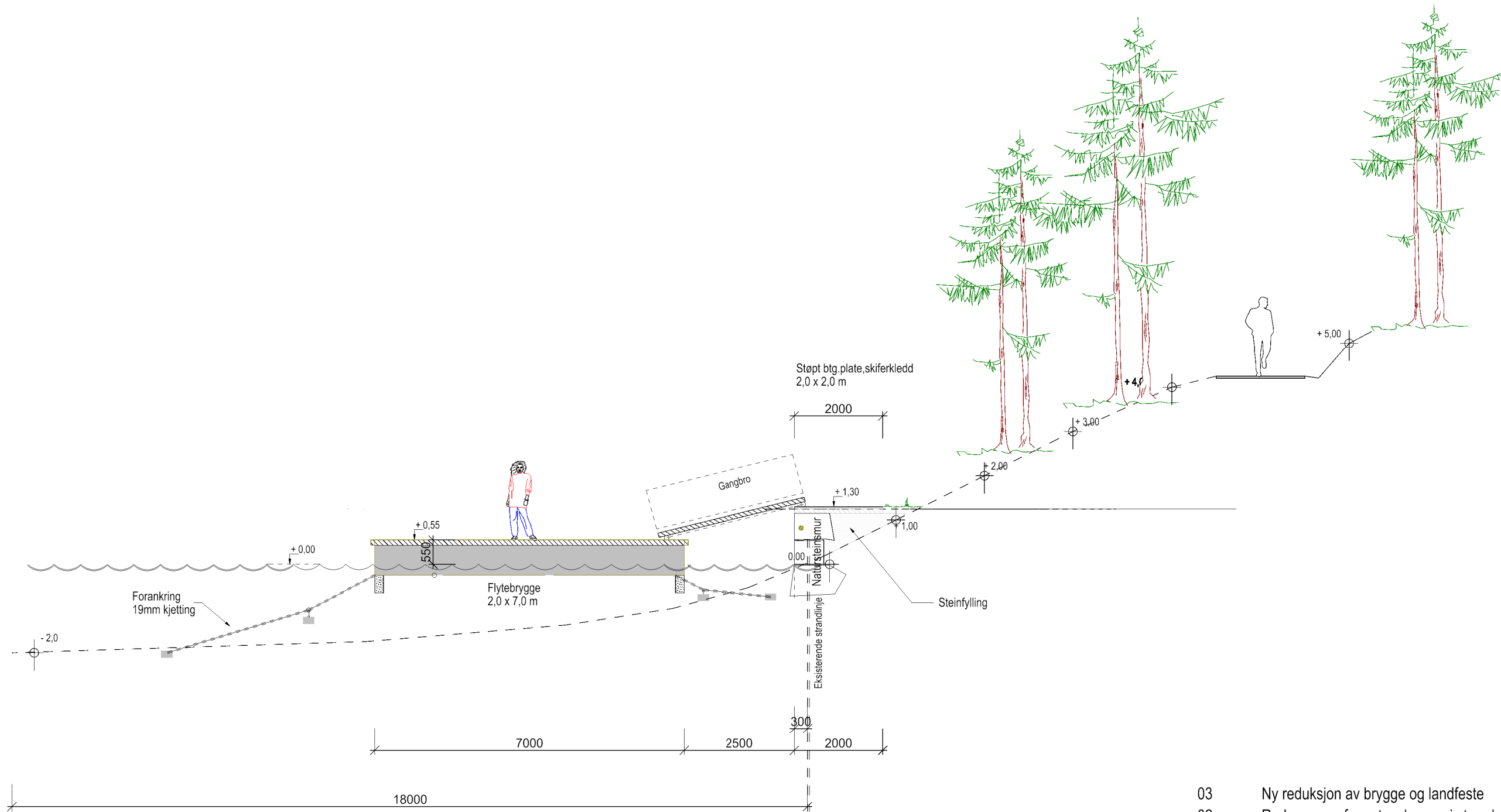
Snitt A-A
