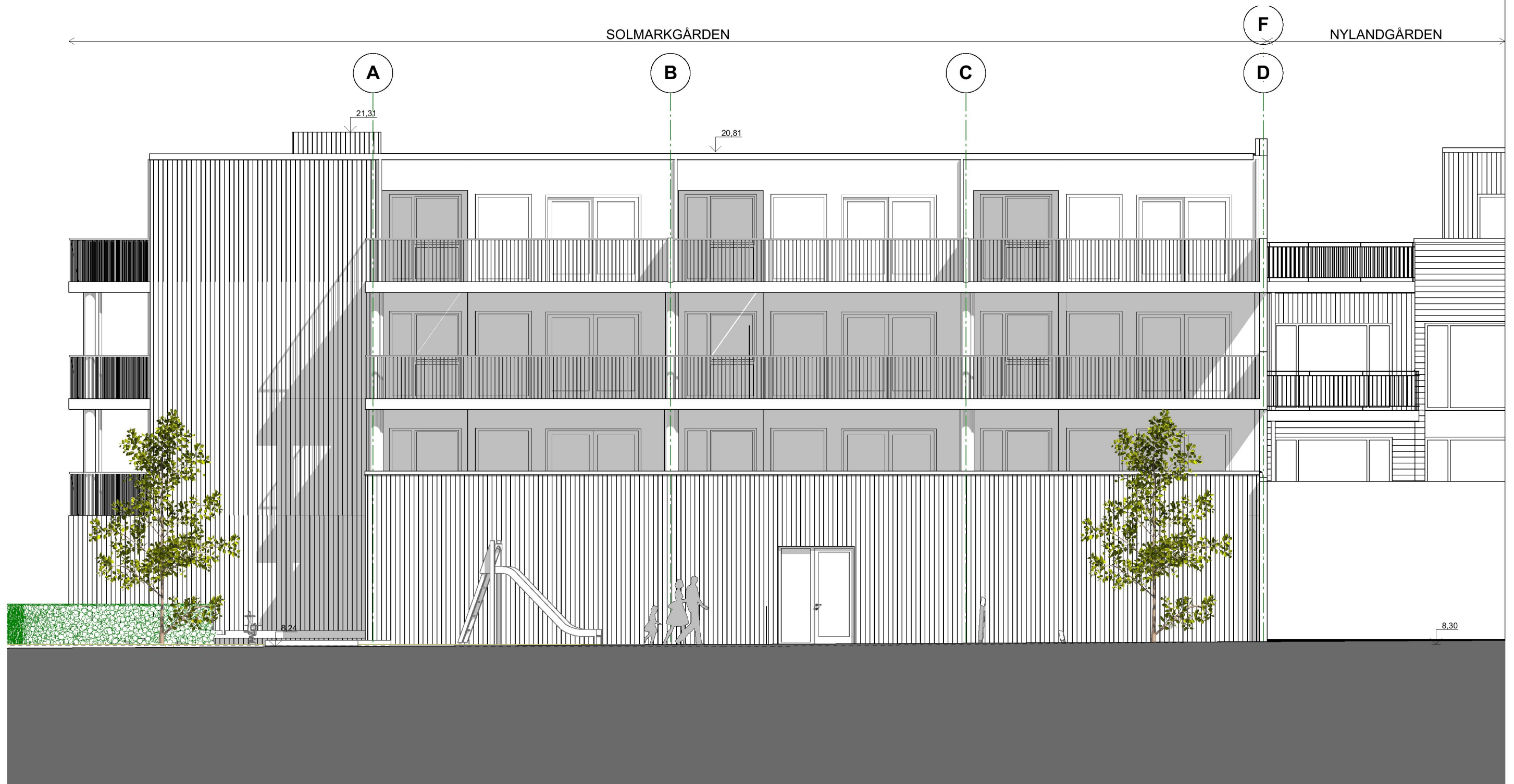
1:100 Fasade Vest
