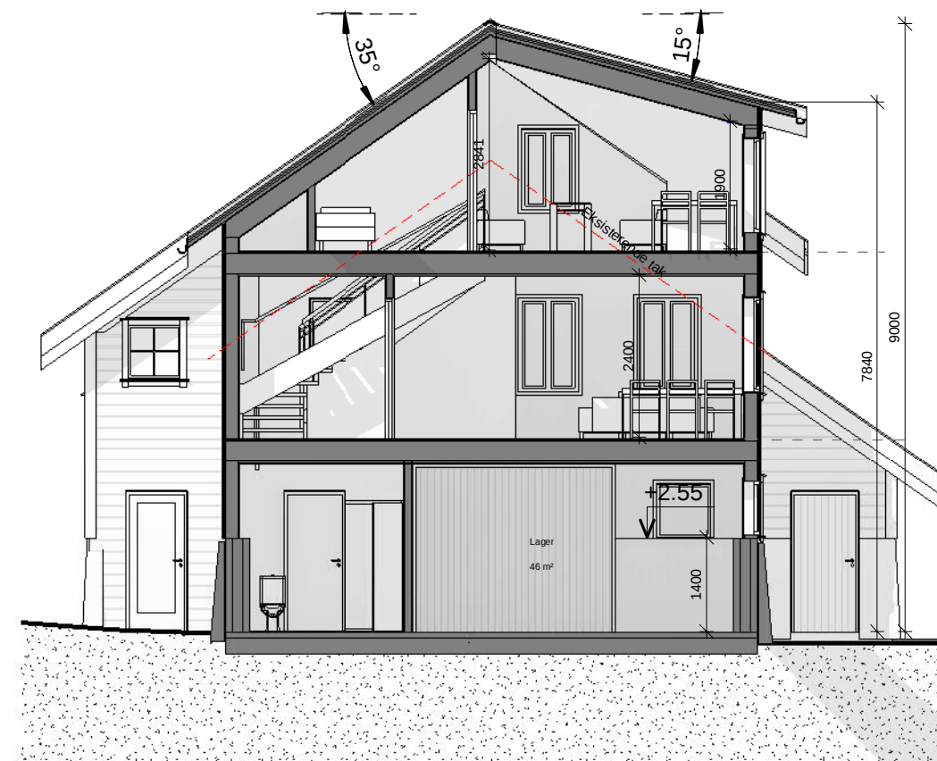
Snitt B-B 1 : 100
