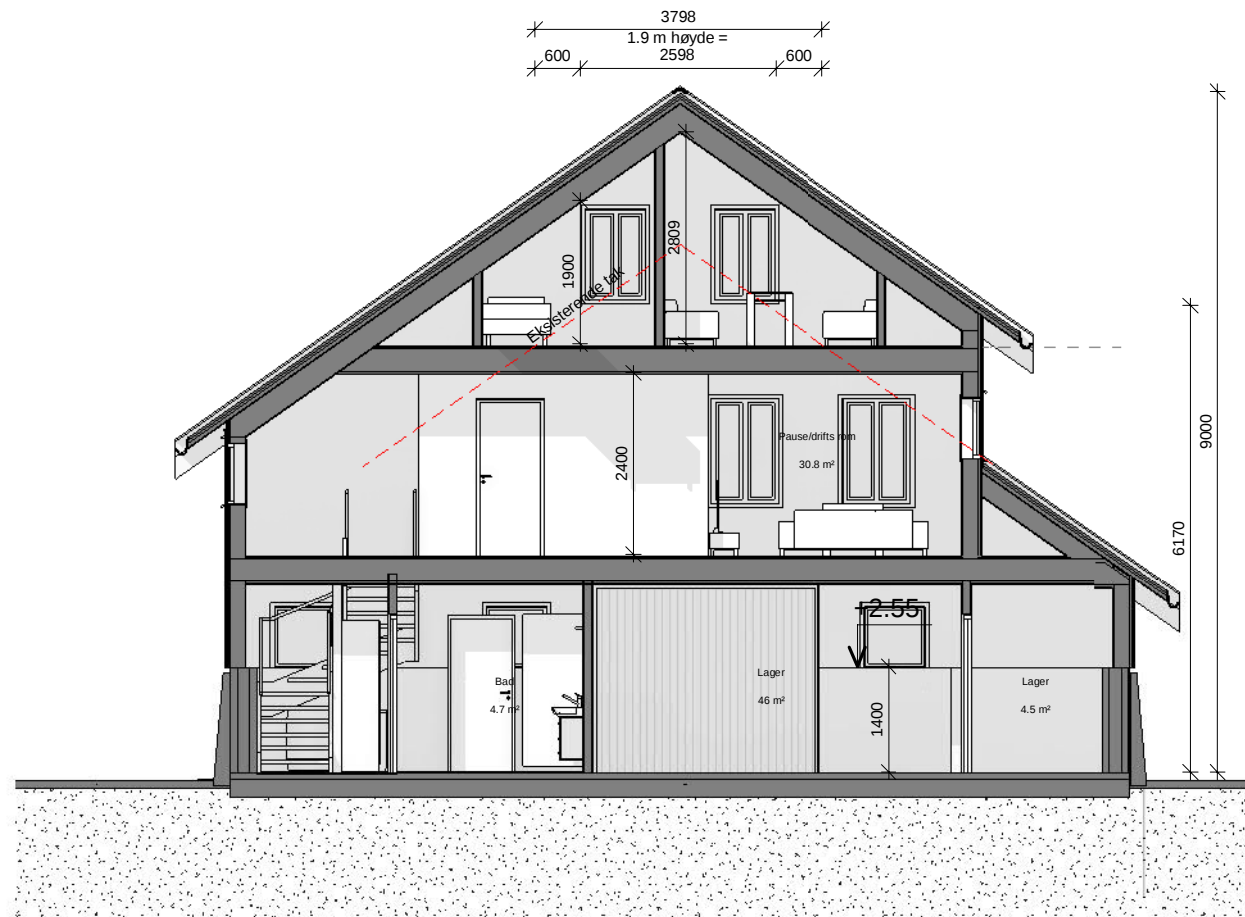
Snitt A-A 1 : 100
