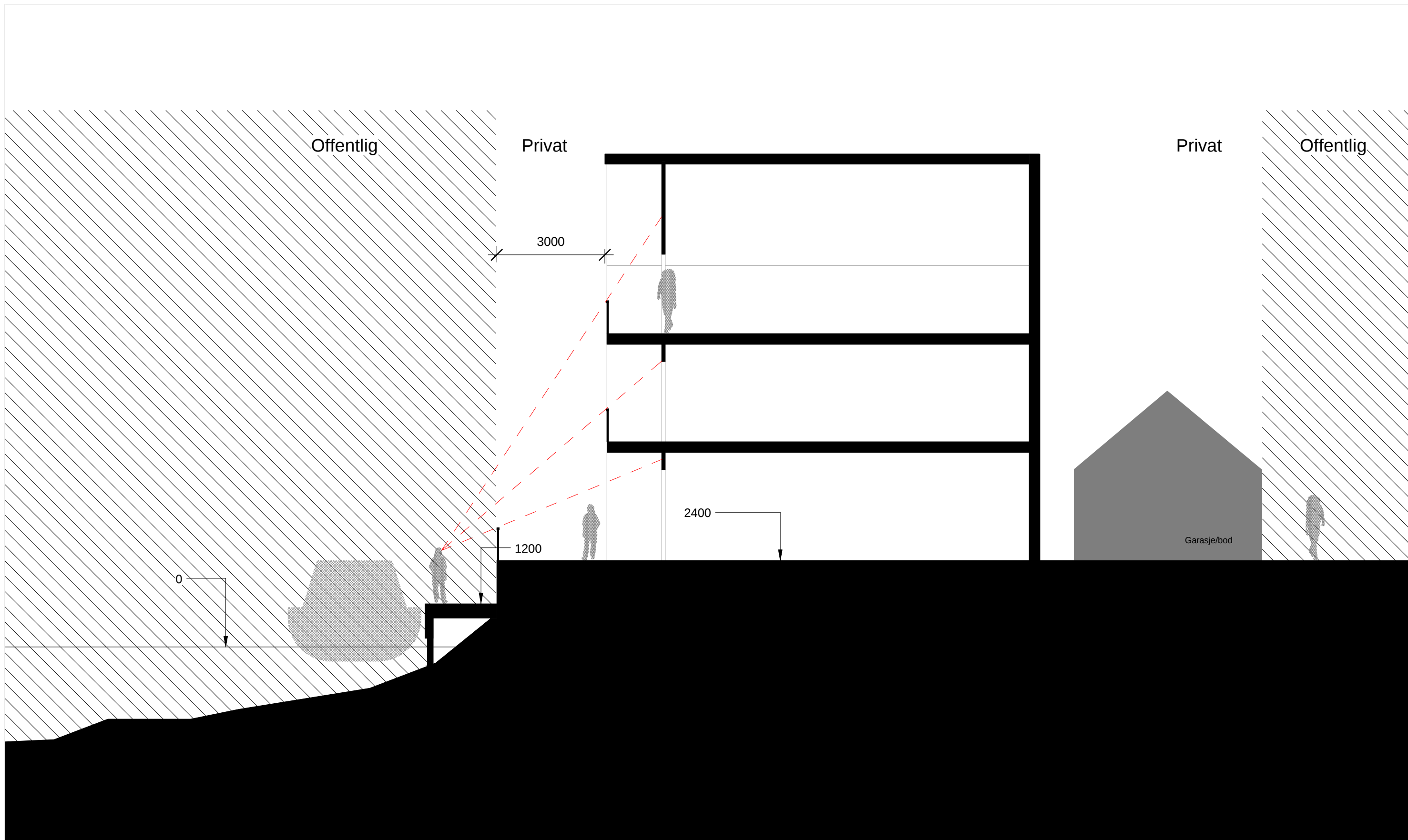
Snitt strandson, A3 1 : 100
